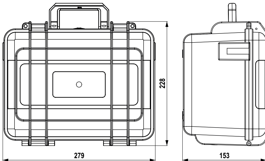
Obr. 1: Rozměry
