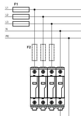
TN-S
