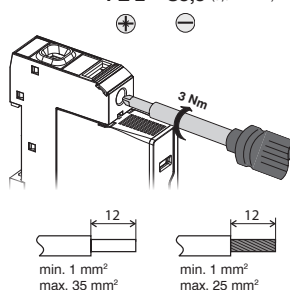
PZ 2 S5,5 (5,5x1 mm)
