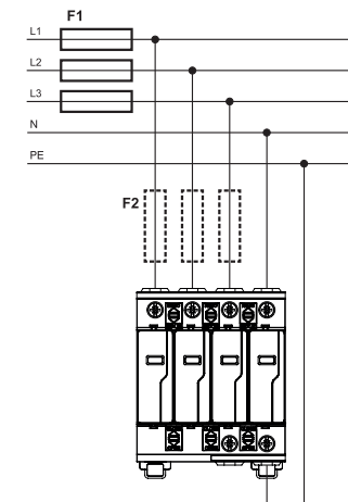
TN-S
