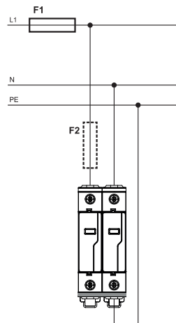
TN-S
