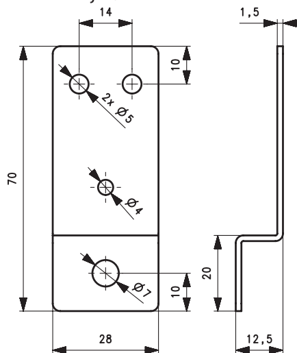
HX-pomocný držák/HX-holder
