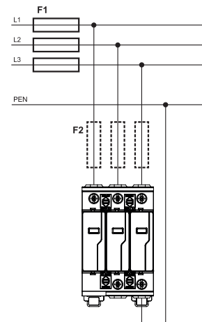
TN-C
