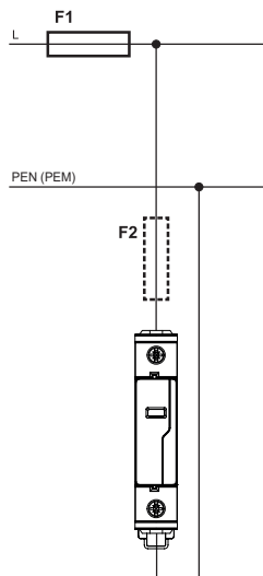
TN-C
