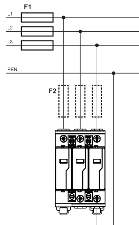
TN-C
