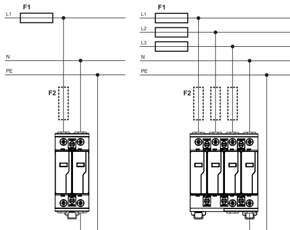
TN-S
