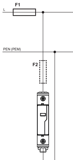
TN-C
