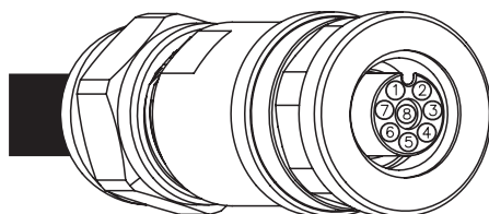
Obr. 8: Připojení konektoru pro datový kabel (Mu - utahovací moment, SW/OK - velikost potřebného klíče)
